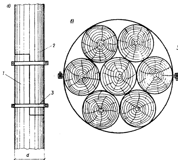
Рис. 16. Установка хомутов
