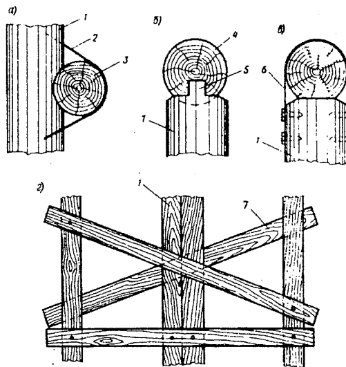
Рис. 15. Установка деревянных элементов
