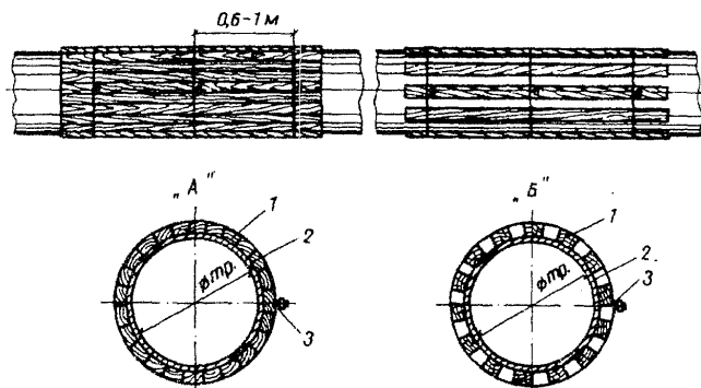
Рис. 6. Футеровка трубопровода деревянными рейками Сечение трубопровода: А - при сплошной футеровке, Б - при несплошной футеровке
