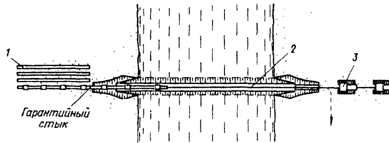
Рис. 8. Схема протаскивания с последовательным наращиванием трубопровода
