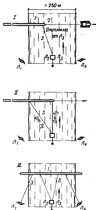
Рис. 10. Схема установки трубопровода в створ при ширине реки более 250 м
