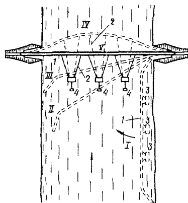
Рис. 11. Схема установки трубопровода в створ разворотом на плаву
