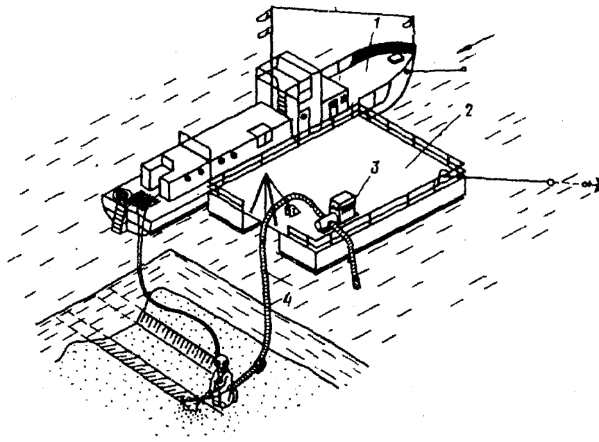
Рис. 3. Схема разработки грунта гидромонитором
